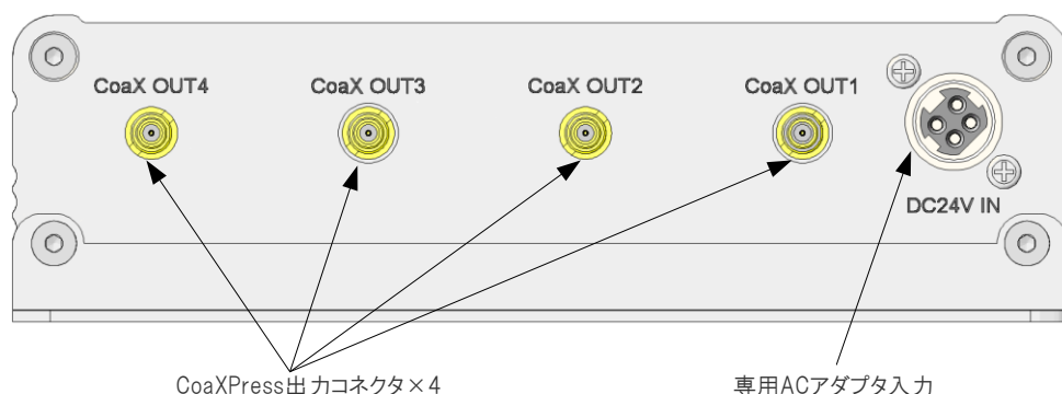
CXR12-400 出力側パネル
