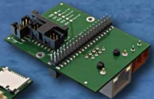
アダプターボード #2
