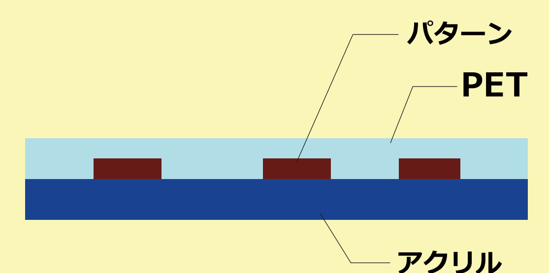
製品構成図
