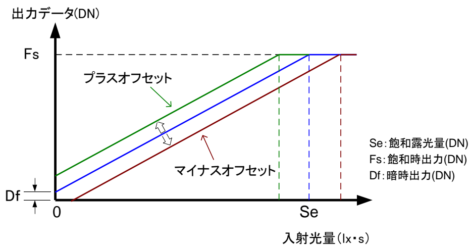
図 4-9-1 オフセットの調整
