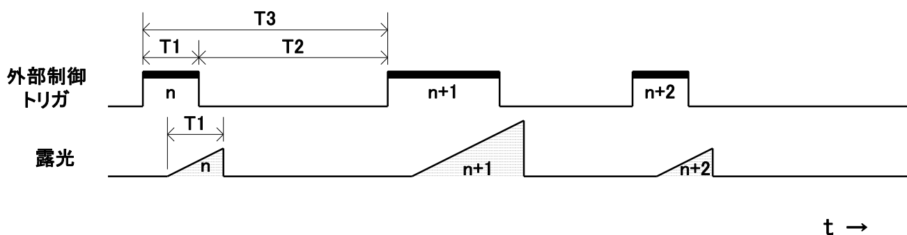
図 4-7-3-1 外部トリガレベルモード
