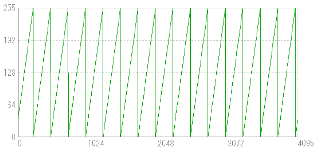
図 4-10-4-5 Mono8 の水平垂直ランプパターンライン波形
