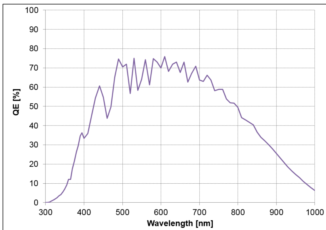
図 1-4-2 量子効率
