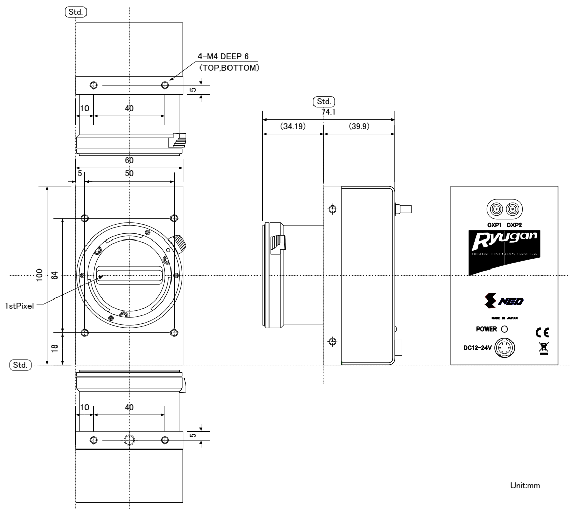
図 2-3-1 外形寸法図 (Fマウント)
