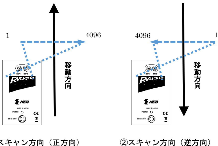
図 4-10-2 移動方向とスキャン方向
