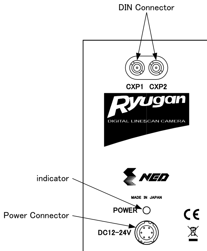
図 3-2-1 コネクタの配置 (Camera Link コネクタ、電源、インディケータ)
