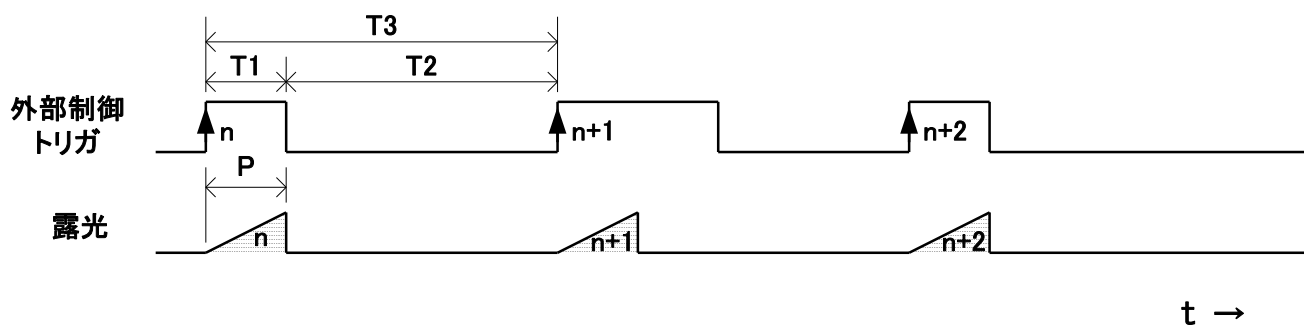
図 4-7-2-1 外部トリガエッジモード
