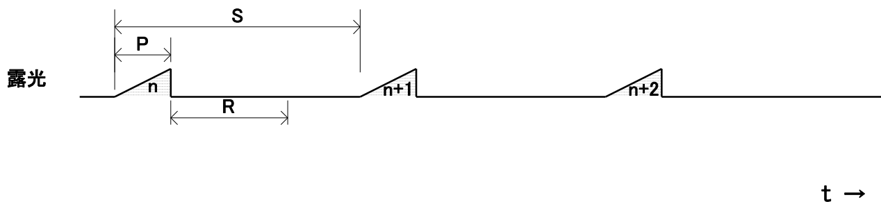
図 4-7-1-1 フリーランモード
